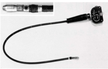
V型胃カメラ。1960年より市販され広く使われた。外径11・7mm。
